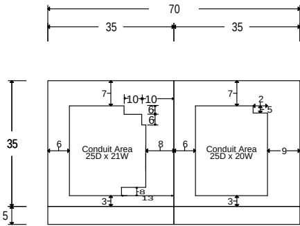
Bottom Conduit Area
