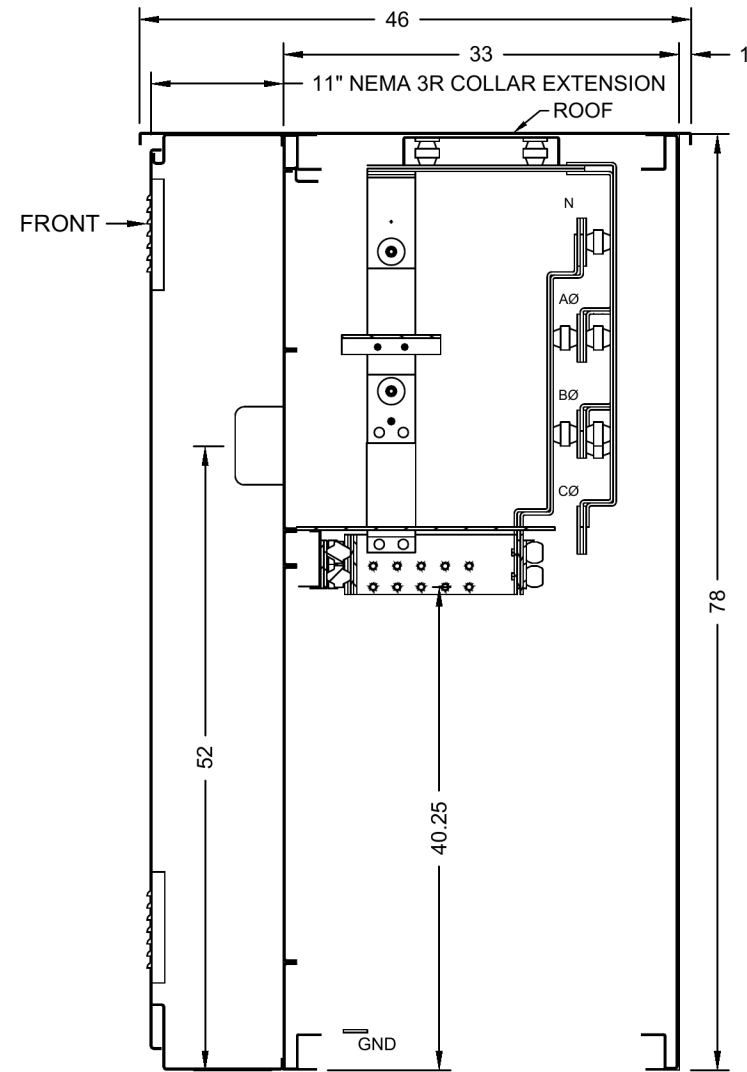
SECTION A-A
